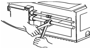
Tubería de cobre aceite aplicado (para reducir fricción con la tuerca
